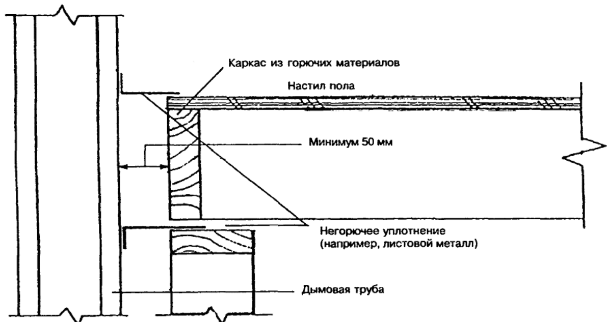
Рисунок 7.8 - Расстояние от дымовой трубы до строительных конструкций
