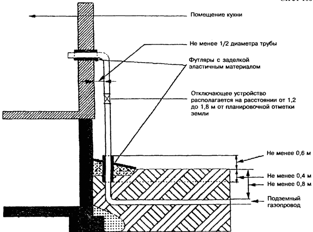
Рисунок 9.1 - Газовый ввод
